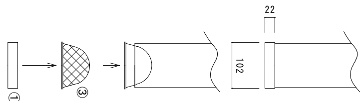
吸込口取付要領
