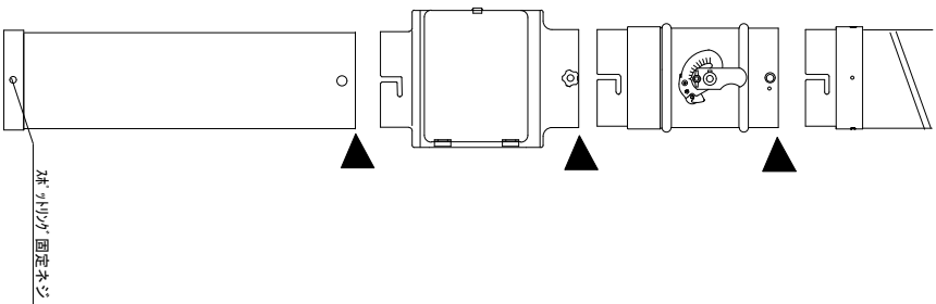
取外し位置詳細図
