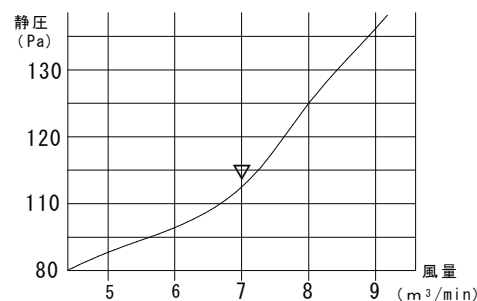
性能特性表
