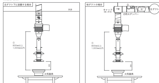
図面詳細図
