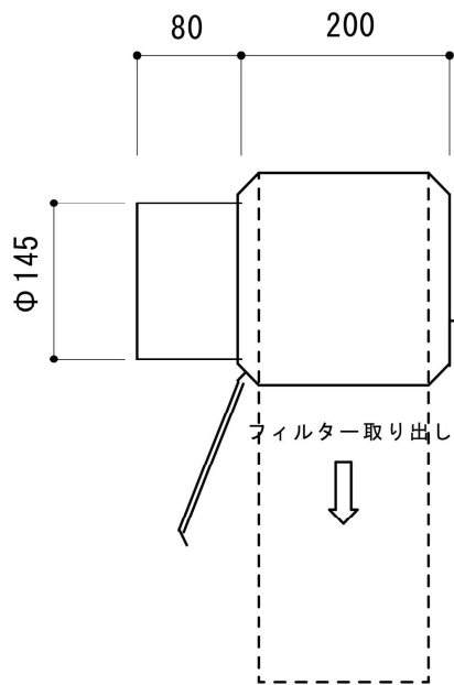
{ フィルターユニット平面図 }
