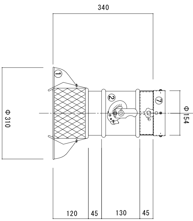
フィルターユニット部 詳細図
